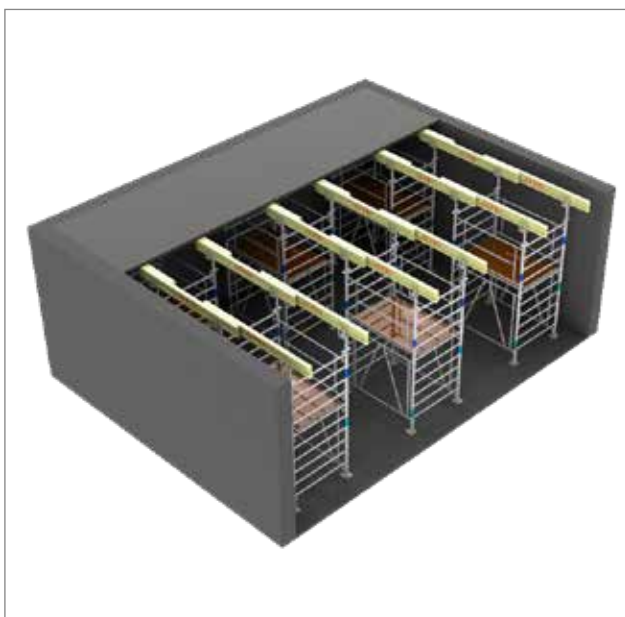
- Étalement de prédalles avec poutrelles H20 sur tours A120.
